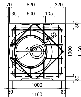
標準組立図 S=1:30
