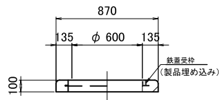
製品構造図
