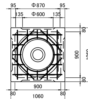
標準組立図
