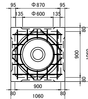
標準組立図 S=1:30
