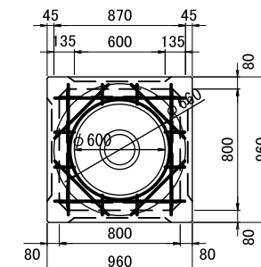
標準組立図 S=1:30
