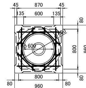
標準組立図
