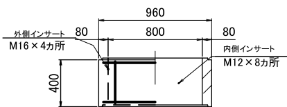
中間400H
